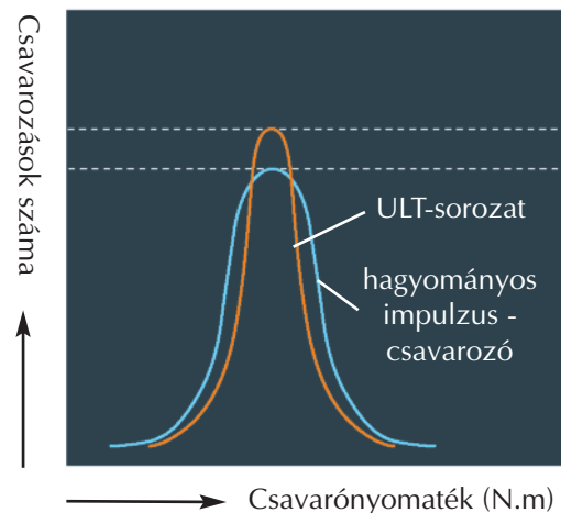
Csavaró-nyomaték - szórás
