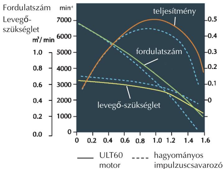
Motoradatok összehasonlítása
